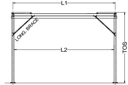
LONGITUDINAL VIEW
